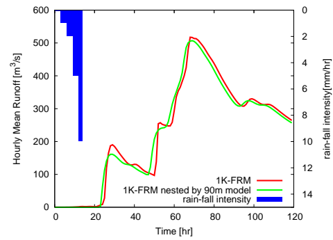
図3 流量(赤:1K-FRMの結果、緑:1K-FRMの結果を領域Aをネスティングした結果、青:降雨強度)
