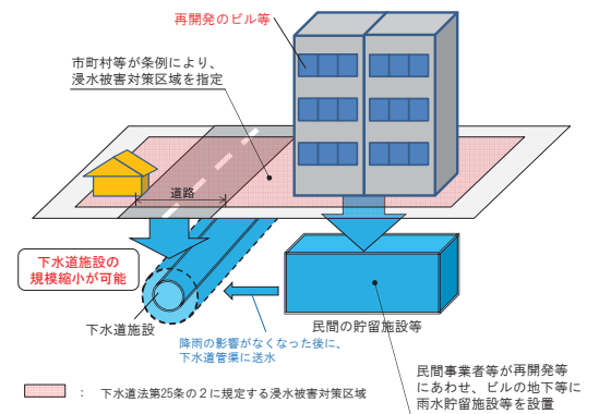
民間の雨水貯留施設を活用した浸水対策
